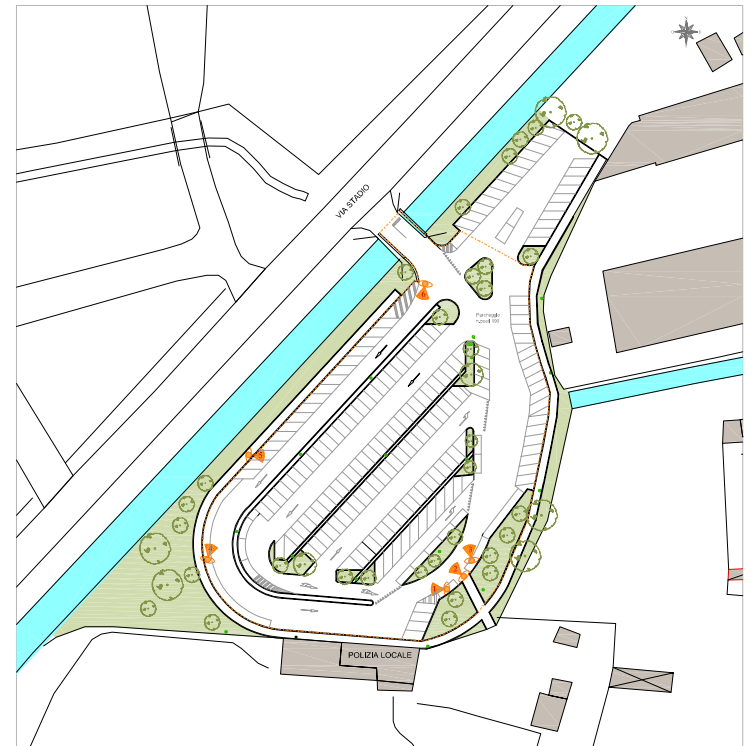
PLANIMETRIA GENERALE - PARCHEGGIO PIAZZA CASTELLO
